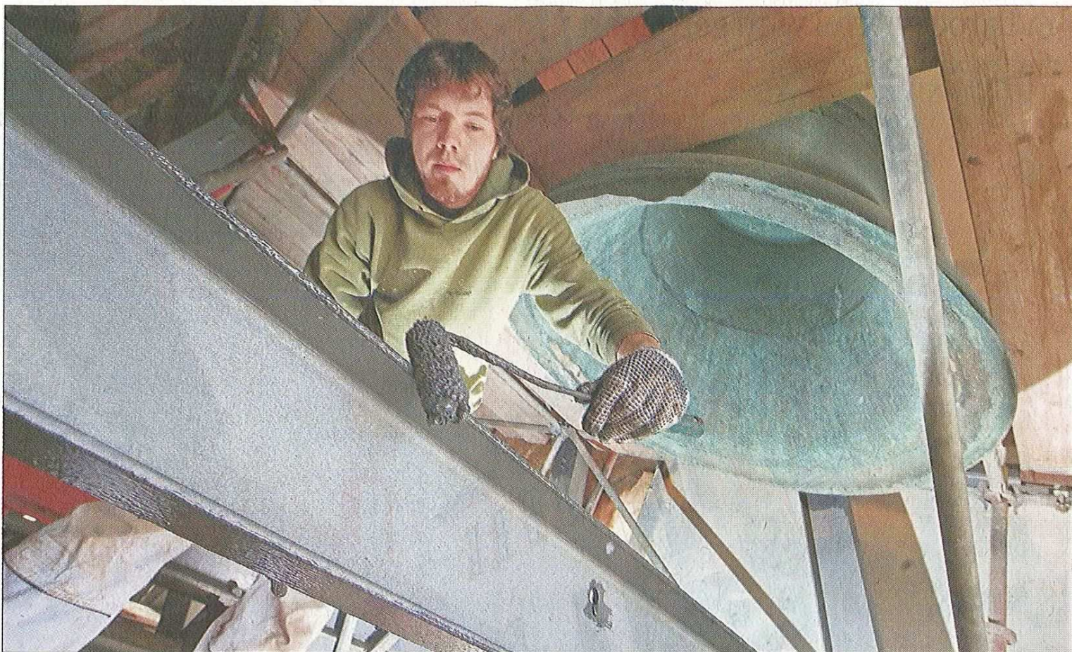
Nachdem der Glockenstuhl mit einem Korrosionsschutz behandelt worden ist, verpasst Maler und Lackierer Thomas Matka von der Dresdner Firma Fuchs & Girke dem Stahl jetzt den letzten Anstrich.
